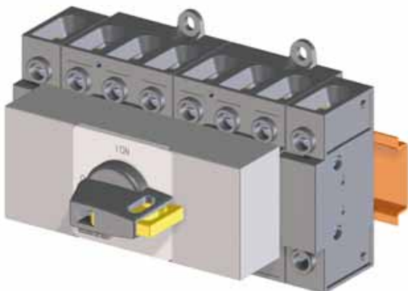
8-poliger Ein-/Ausschalter
